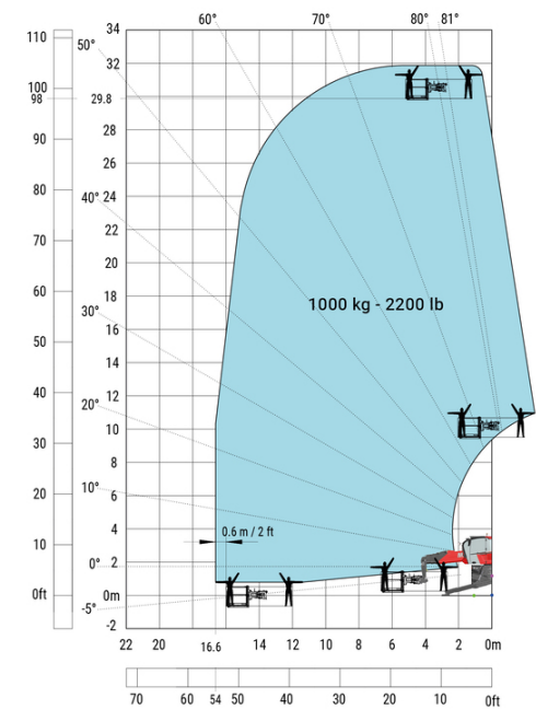
Rotazione su stabilizzatori con cestello da 1000 kg
