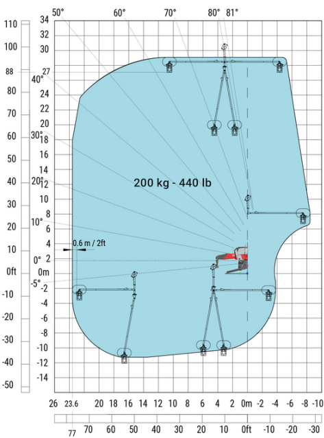
Rotazione su stabilizzatori con cestello 3D negativo
